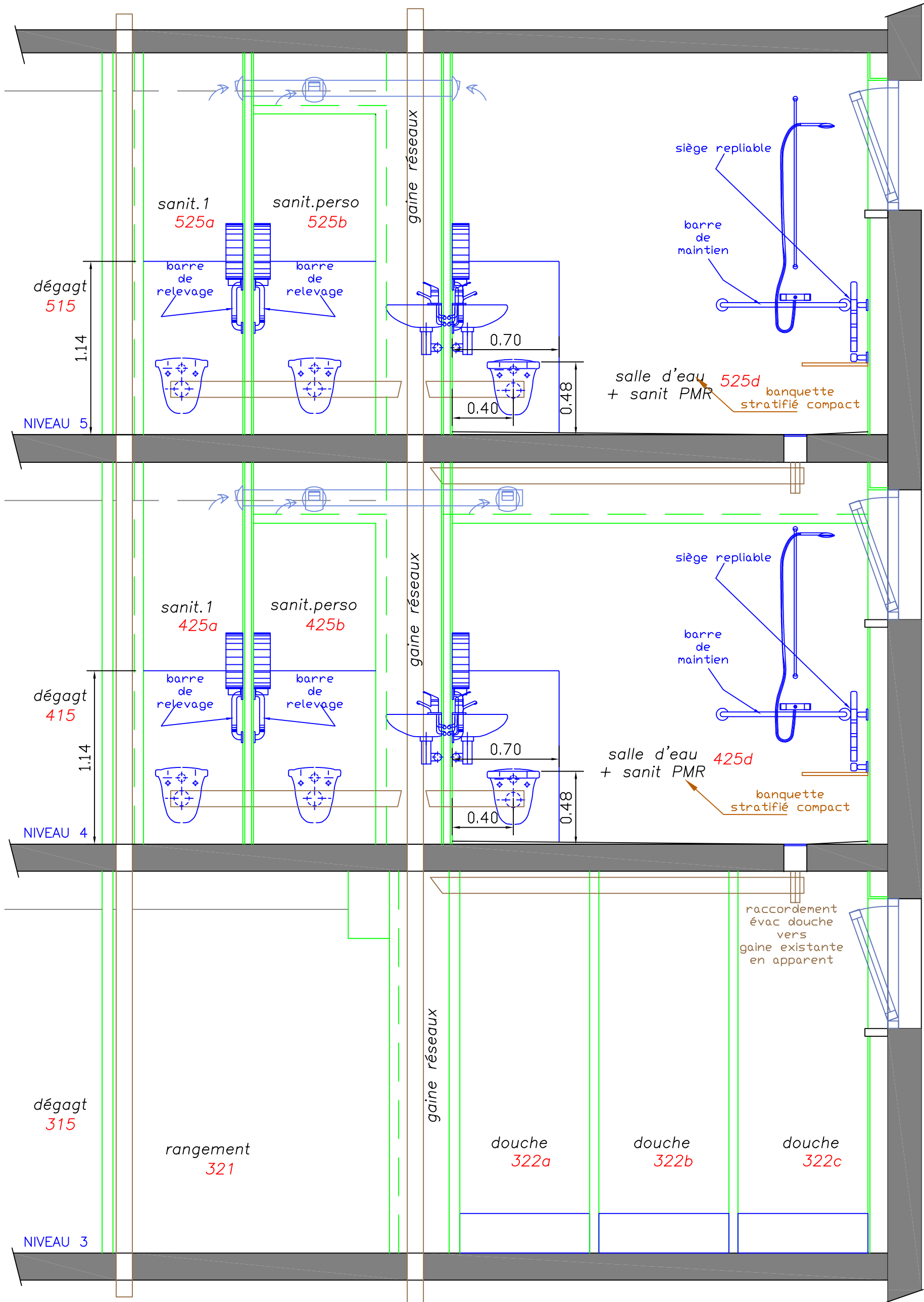
COUPE DD gpes 2&4
