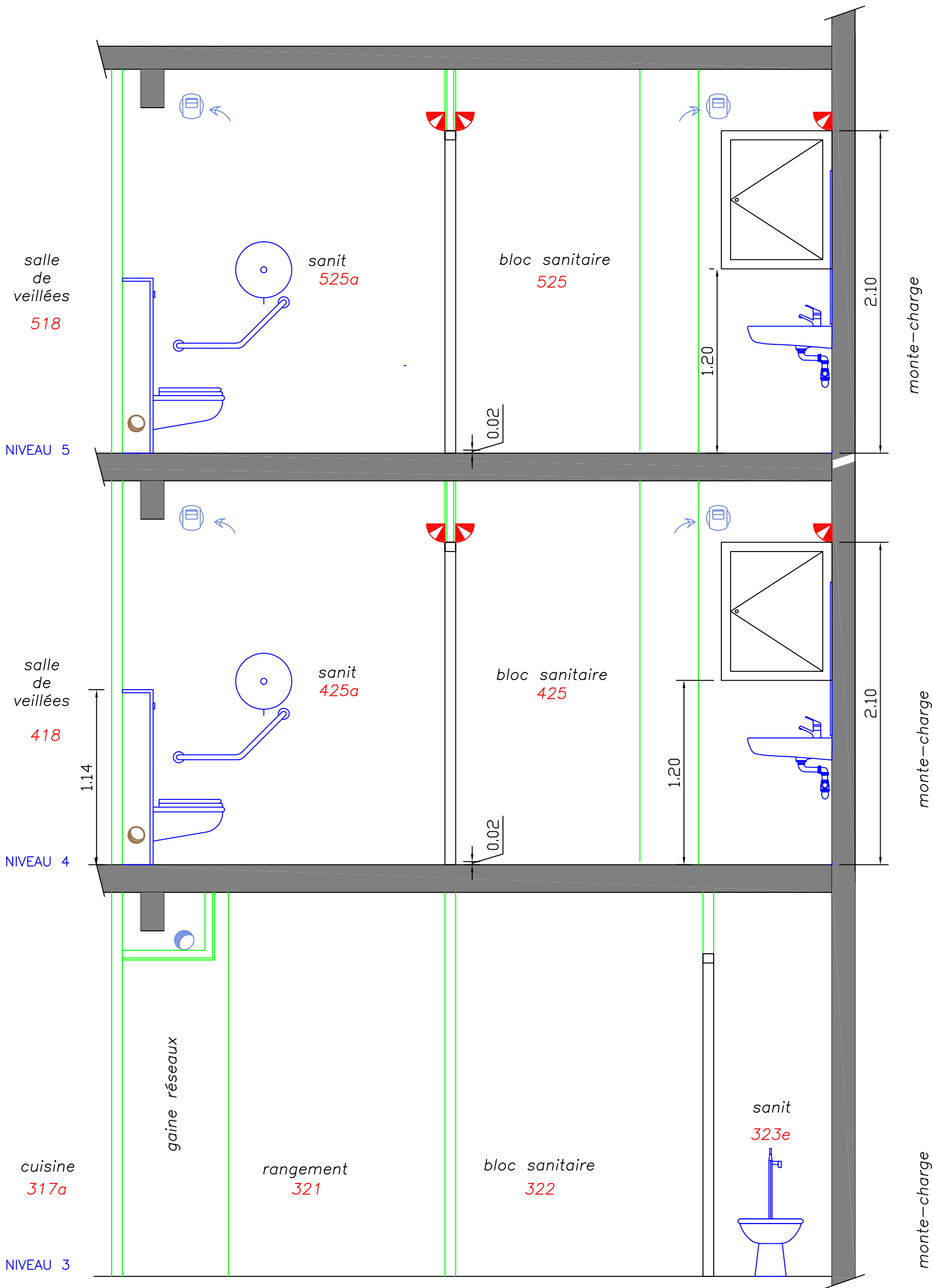
COUPE CC gpes 2&4
